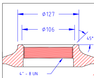
Détail Filetage 4"
