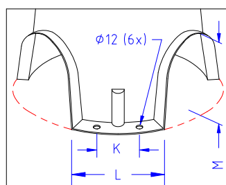
DÉTAIL SOCLE
