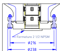
DÉTAIL BRIDE DE 6"
