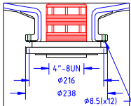
DÉTAIL SUPÉRIEUR/ INFÉRIEUR BRIDE DE 6"
