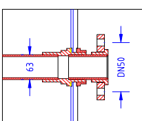
DÉTAIL ORIFICE LATÉRAL
