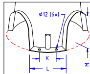
DÉTAIL SOCLE
