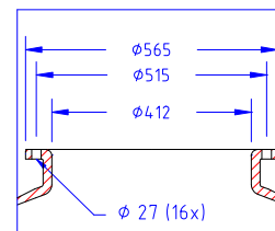
DÉTAIL BRIDE SUPÉRIEURE DE DN400
