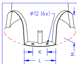
DÉTAIL SOCLE
