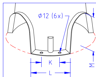
DÉTAIL SOCLE
