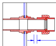
DÉTAIL ORIFICE LATÉRAL
