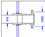
DÉTAIL DN80
