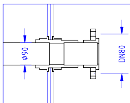
DÉTAIL DN80
