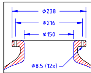
DÉTAIL BRIDE DE 6"
