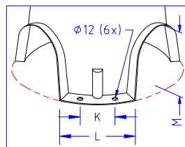
DÉTAIL SOCLE
