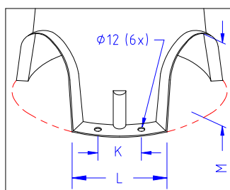
DÉTAIL SOCLE
